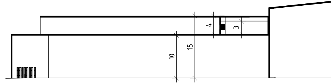
SEKTION A 1:500 (A3)
